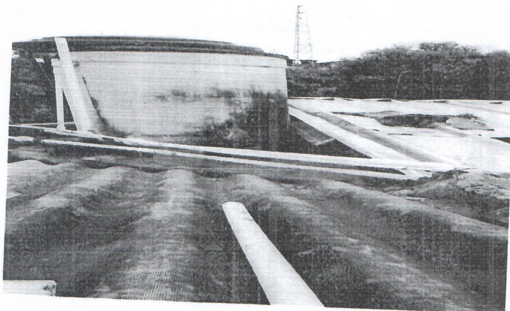
Foto No. 06 Fecha: mayo de 2018 Lugar: Neiva – Huila Obra: Remodelación casa de habitación Descripción: Fugas tubería tanque de almacenamiento
