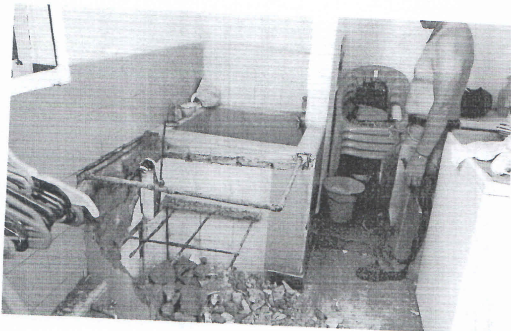
Foto No. 10 Fecha: mayo de 2018 Lugar: Neiva – Huila Obra: Remodelación casa de habitación Descripción: Lavadero y tanque con fugas de agua
