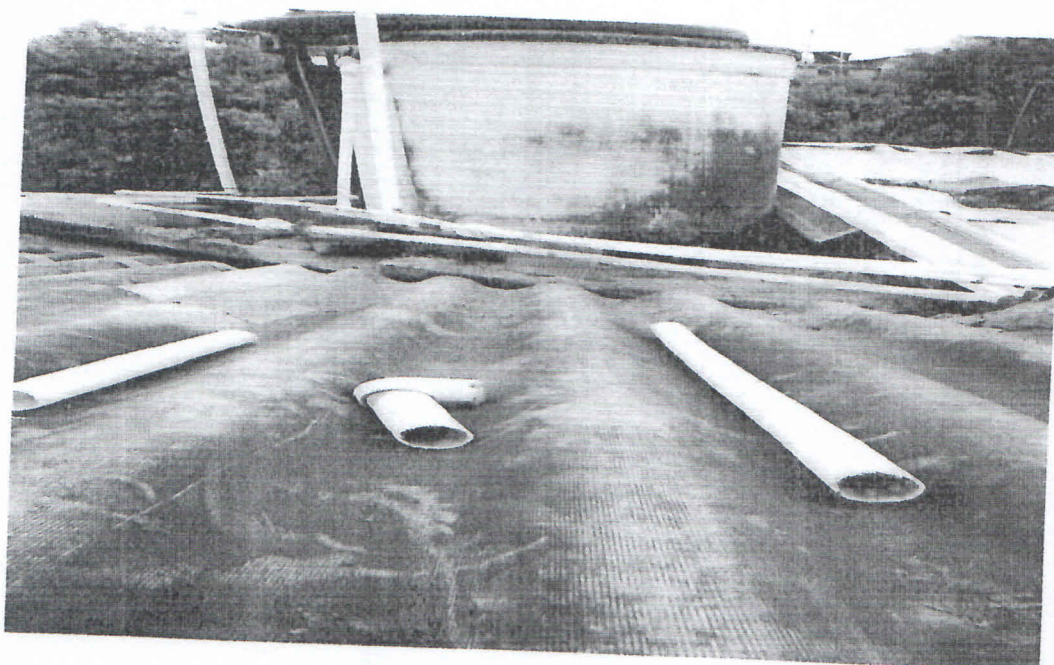
Foto No. 05 Fecha: mayo de 2018 Lugar: Neiva – Huila Obra: Remodelación casa de habitación Descripción: Fugas tubería tanque de almacenamiento
