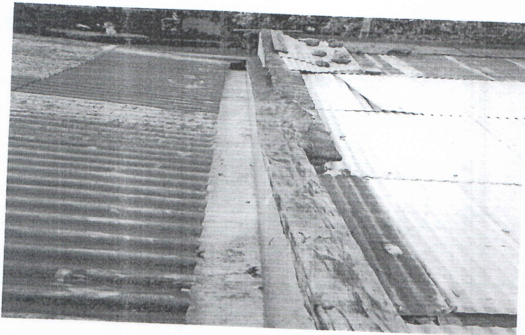
Foto No. 07 Fecha: mayo de 2018 Lugar: Neiva – Huila Obra: Remodelación casa de habitación Descripción: Fugas canal para recolección aguas lluvias
