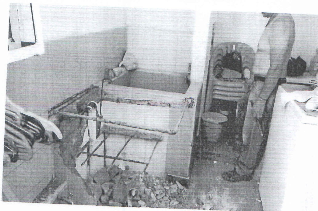
Foto No. 10 Fecha: mayo de 2018 Lugar: Neiva – Huila Obra: Remodelación casa de habitación Descripción: Lavadero y tanque con fugas de agua
